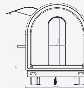
FACE ARRIÈRE
